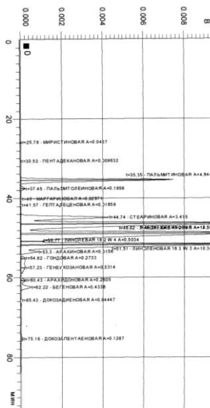
Рис. 1. Хроматограма лляної олії
