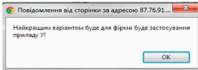
Рис.3.8. Діалогове вікно
